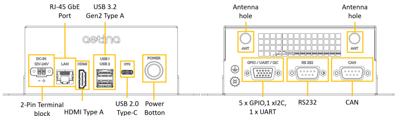
Figure 2.1 AIE-KO21/AIE-KO31/AIE-KN31/AIE-KN41 I/O Interface
